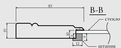
витрина
