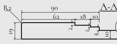
глухой фасад
